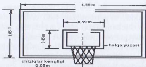
34-rasm. Shitning o'lchovlari.
