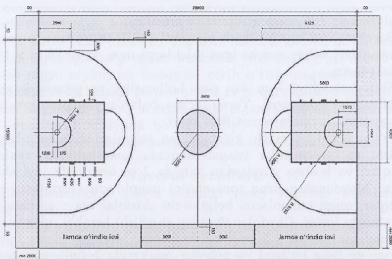
33-rasm. Basketbol maydon o'lchamlari.
